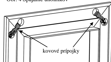
Obr. 4 Spájanie uholníkov
