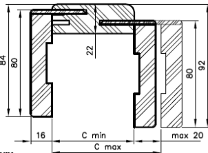
Obr.2 Prierez Tunelu Nastaviteľného s uholníkom T80
