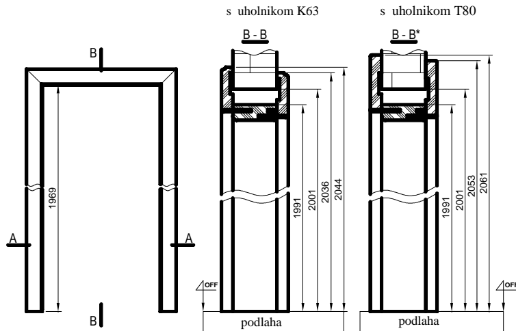
Obr. 6. Podlaha a prierezy Tunelu Nastaviteľného
