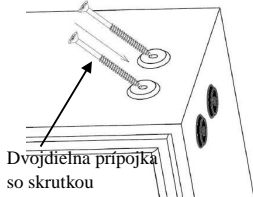
Obr. 3 Spájanie trávov tunelu
