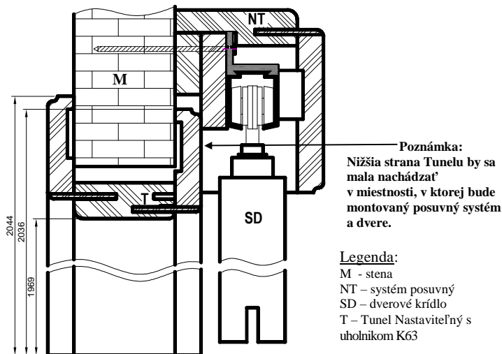
Obr. 9. Využitie Tunelu Nastaviteľného pre systém posuvných dverí NT
